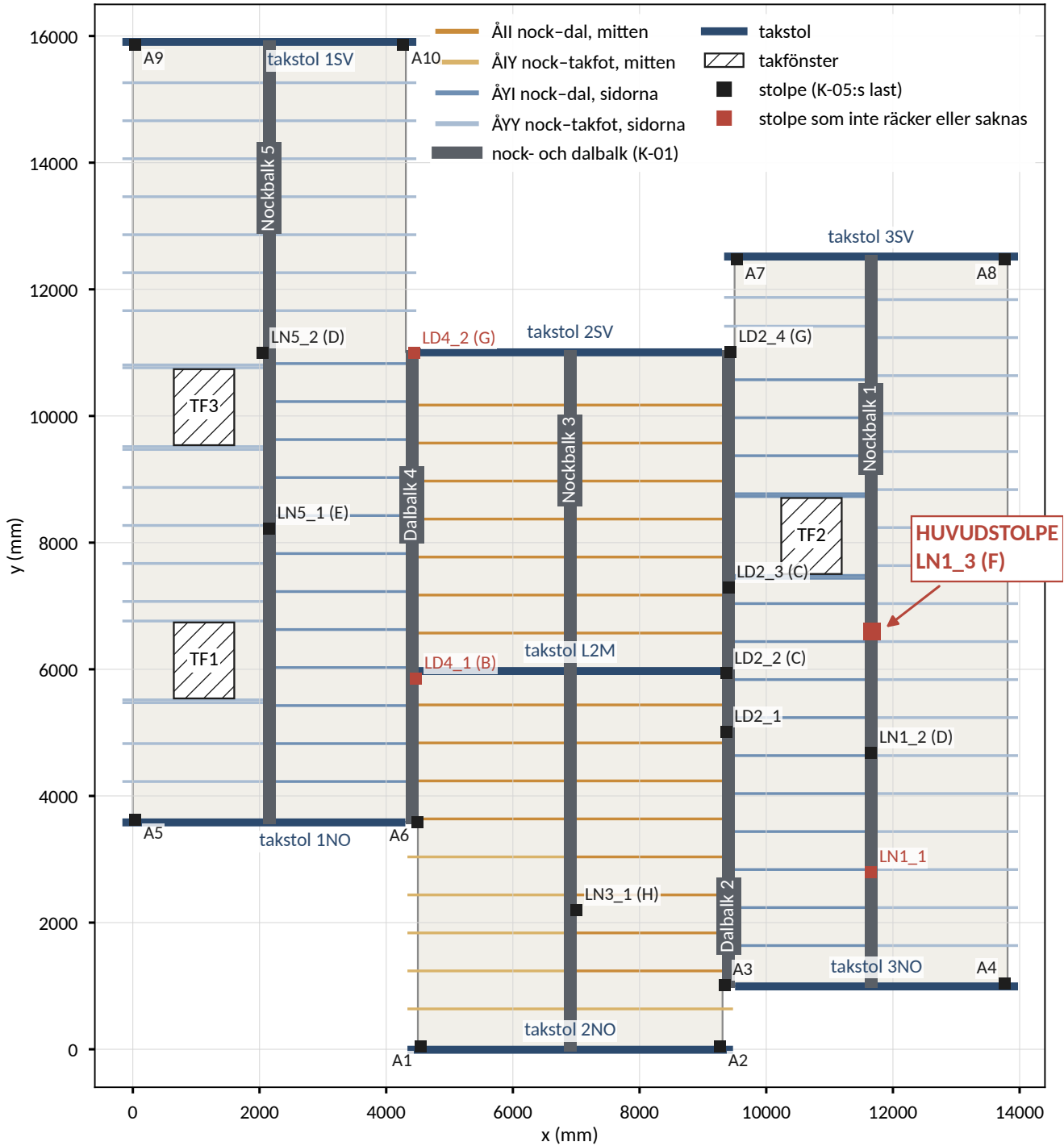
Figur 1: Takets bärande delar i plan, koordinater som i K-05. Röda stolpar räcker inte eller saknas i modellen, se tabellen nedan.
